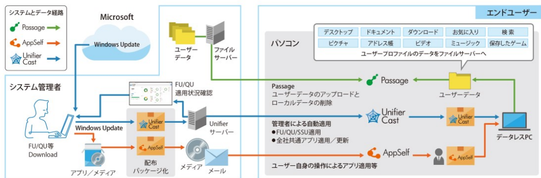
Unifier Cast、AppSelf 導入時の構成イメージ図
