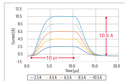
10μs電流出力を15MSa/s サンプリング・レートのデジタイザ・モードで測定
