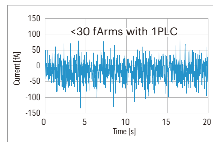
電源測定ノイズ (@ オープン負荷条件)
