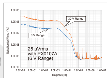
専用フィルタで低ノイズを実現
